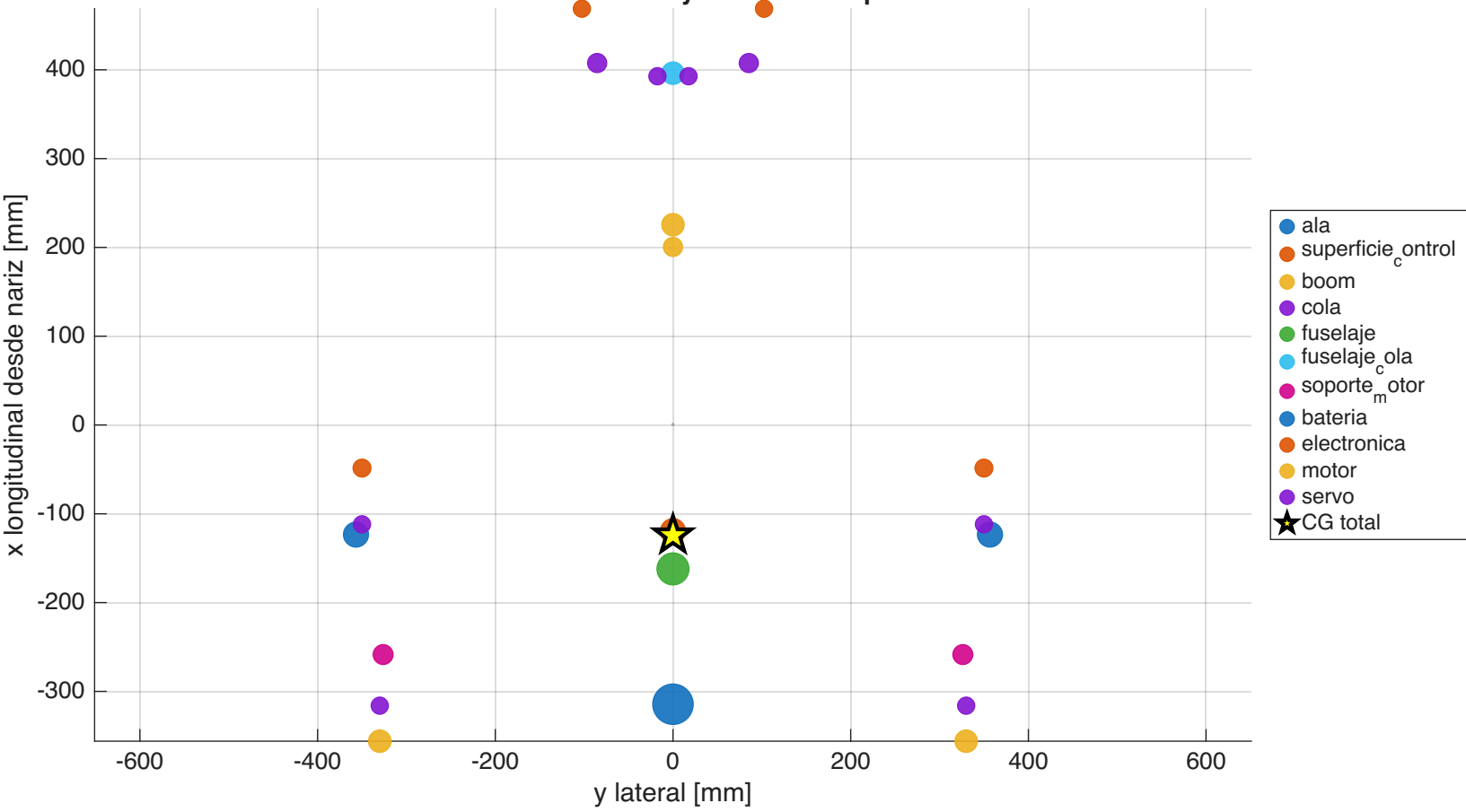
Distribucion de masa y CG - vista superior
